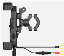
YF-343C-03 连体旋转横杆款
