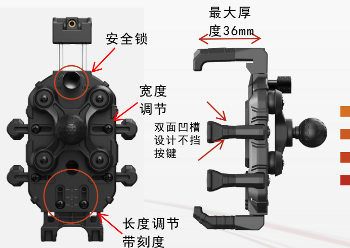
YF-352A-02 连体旋转横杆款
